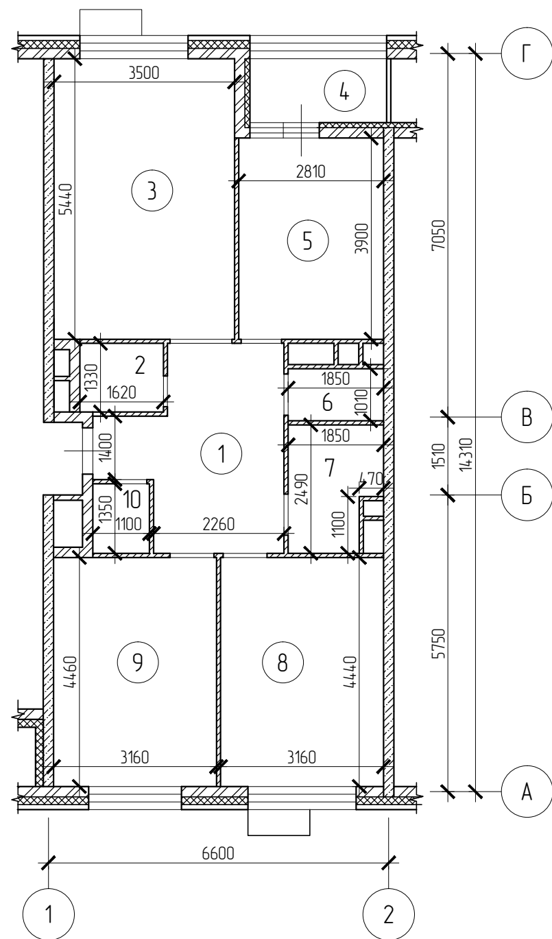
План помещения квартиры до перепланировки и переустройства (М1:100)
