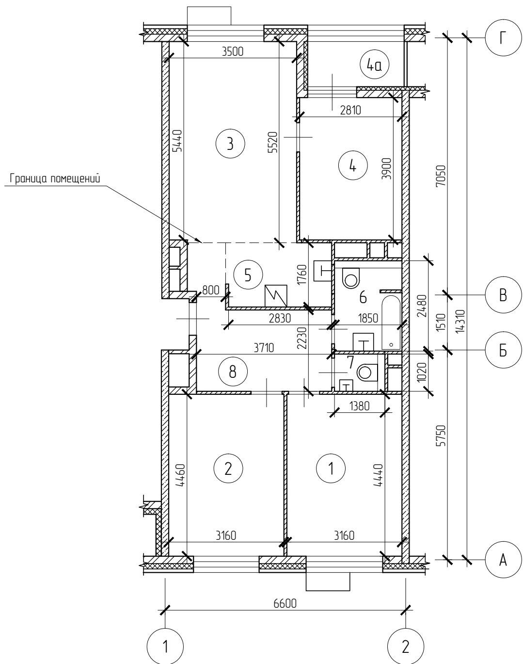
План помещения квартиры после перепланировки и переустройства (М1:100)
